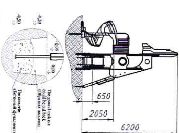
The equipment mounting plan (Схема монтажа оборудования)
