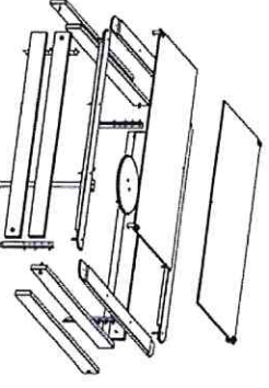
Elements assembling scheme (Общая схема сборки элементов конструкции)
