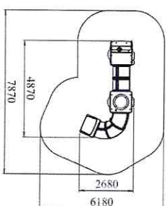
Scheme of the post-planting with foundations (Схема расположения фундамента со столбами)
