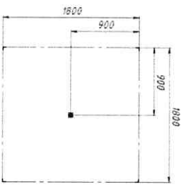
Scheme of the post placing with foundations (Схема расположения фундаментов со столтиками)
